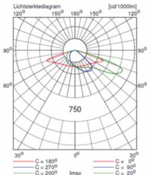
Figuur 14: Lichtsterkediagram
