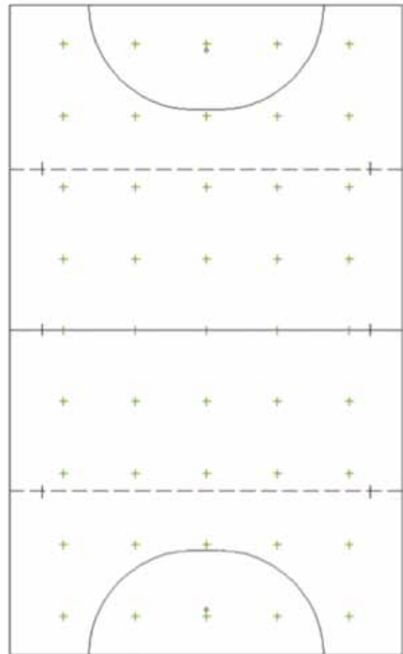
Figuur 18: Meetraaster 10 x 10 meter.
